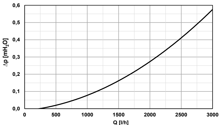
Graf tlakovej straty výmenníka
