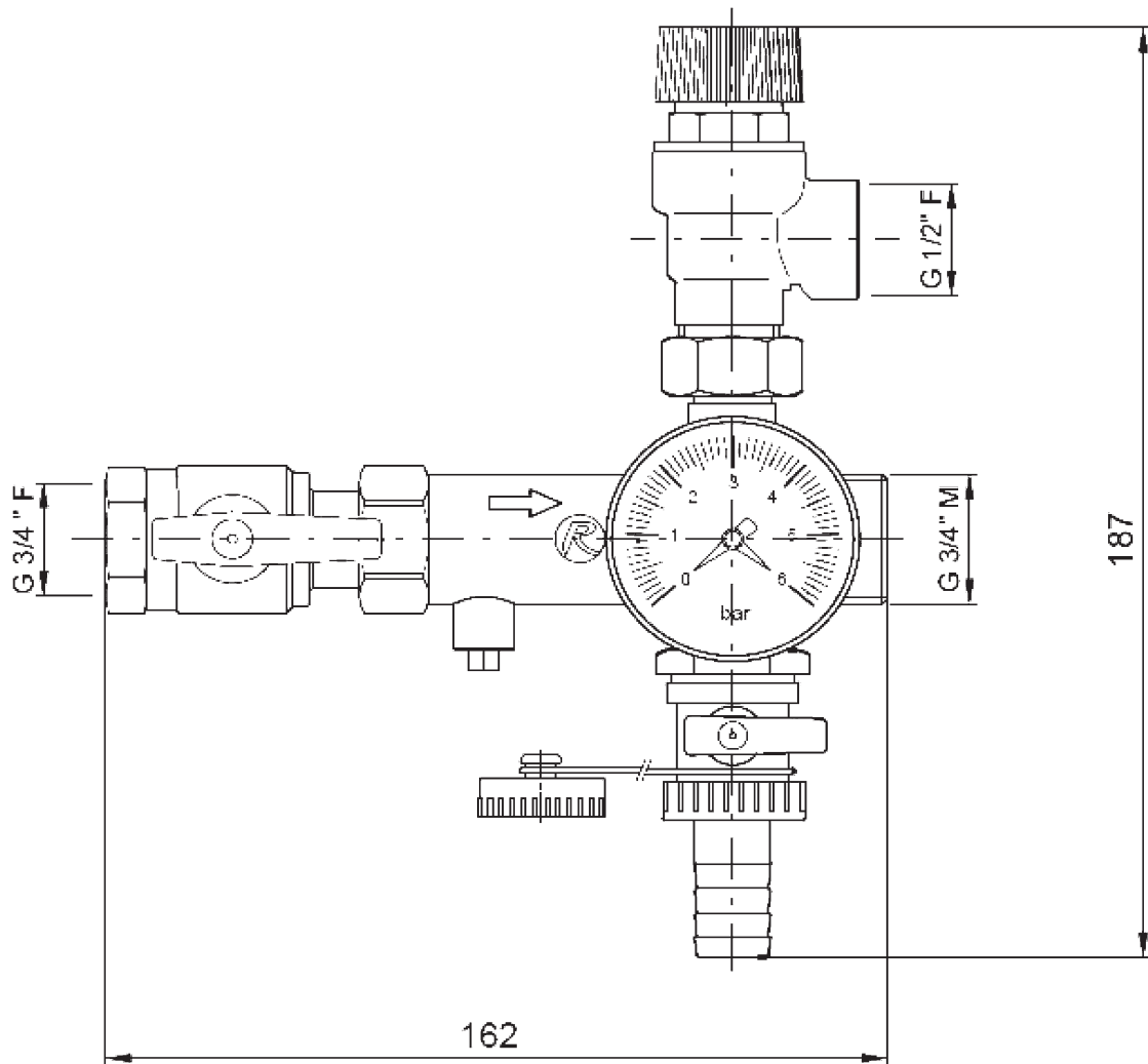
Габаритная схема собранного комплекта
