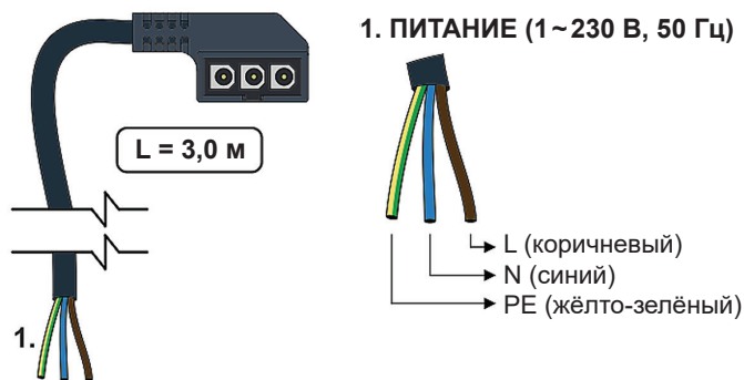
Электрическое подключение насоса
