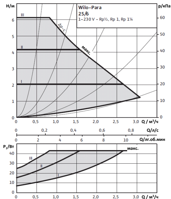
Характеристики Др-с (постоянная)
