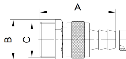
3/4" Сливной кран, без ручки
