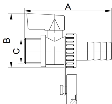
1/2" Сливной кран, с ручкой
