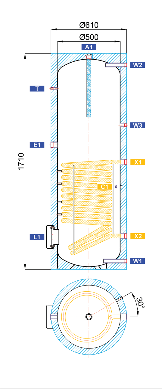
Rozměrové schéma
