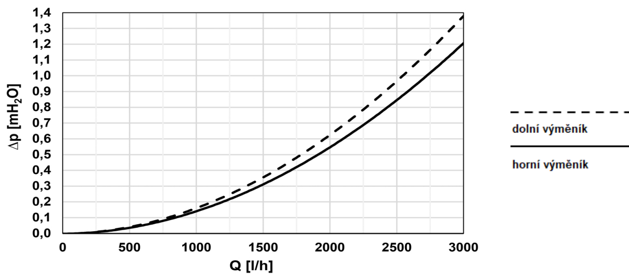
Graf tlakových ztrát
