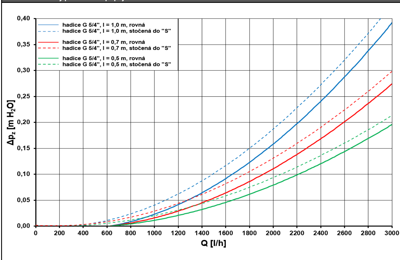
Graf tlakové ztráty pro hadici s přípojením G 5/4"
