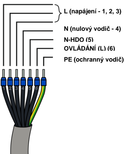
Značení vodičů
