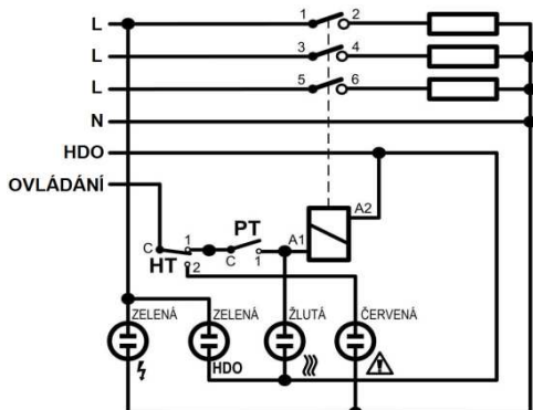
Značení vodičů
