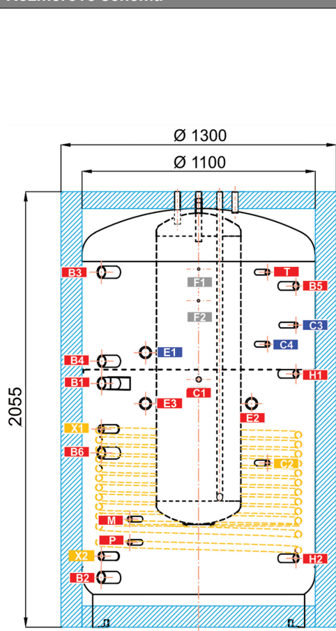
Rozměrové schéma
