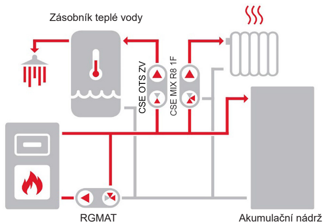
Příklad zapojení I
