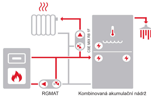
Příklad zapojení II
