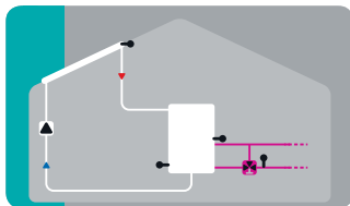
Solárny systém s výmenníkom so špeciálnou funkciou Predohrev spiatocky
