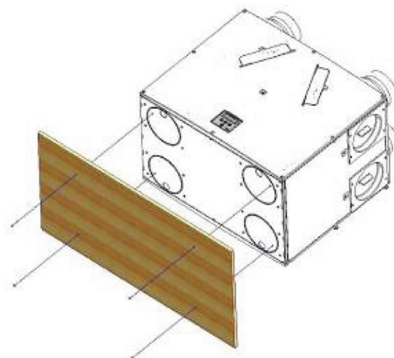
Obr. 19: Upevnění jednotky na podlahu
