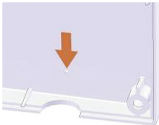
Obr. 12: Vyříznutí 32 mm otvoru pro 22 mm hadici (zadní strana)
