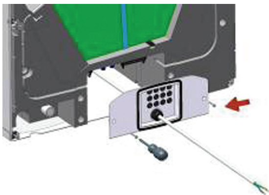
Obr. 6: Odmontování zadní desky s kabelem (zadní strana)
