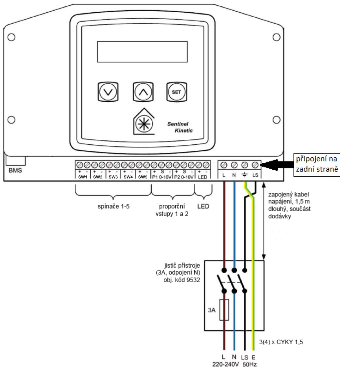
Obr. 21: Zapojení svorek
