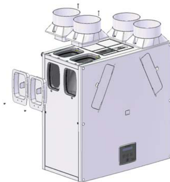
Obr. 16: Demontáž a instalace hrdel
