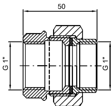
šroubení přímé G 1" F
