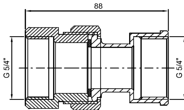
šroubení přímé G 5/4" F
