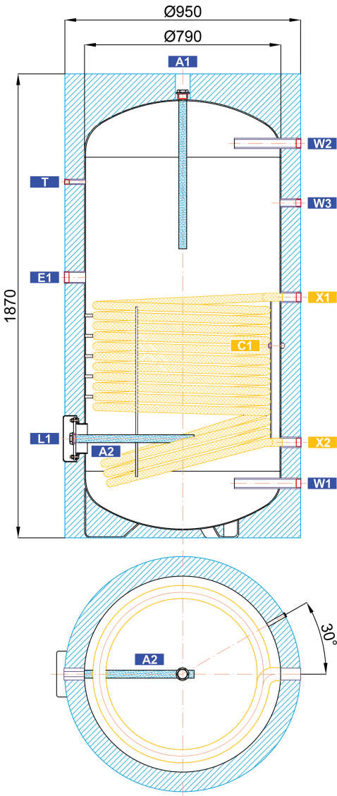
Rozměrové schéma
