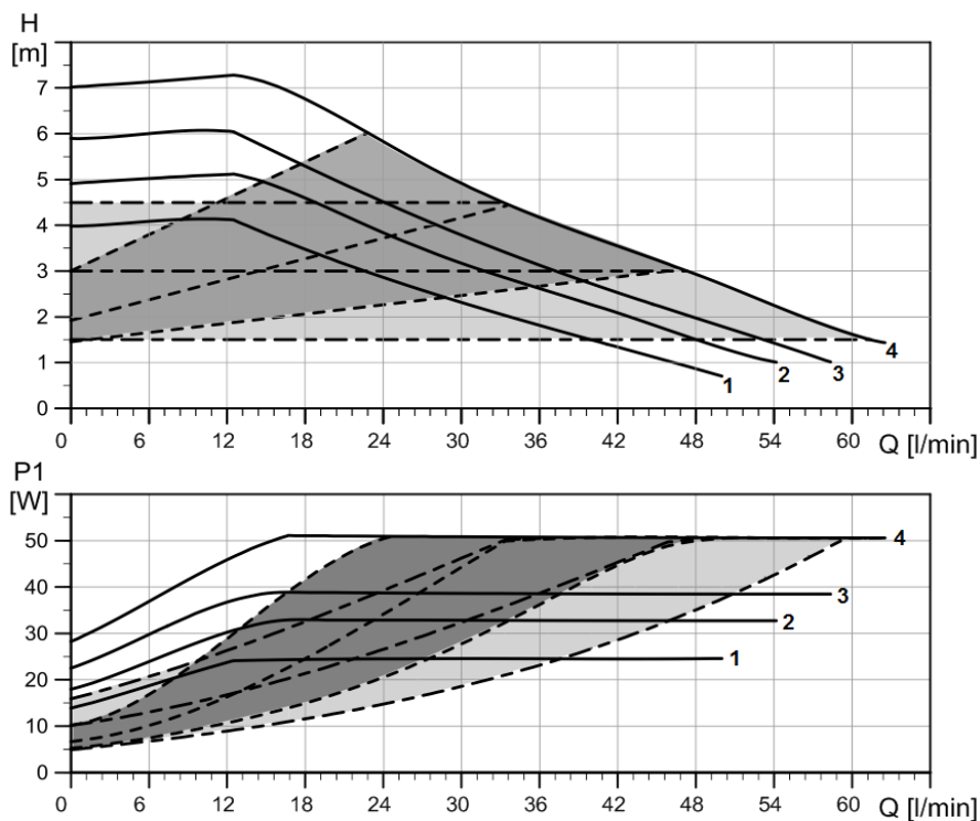
Výkonové krivky čerpadla UPM3 HYBRID 25-75 180
