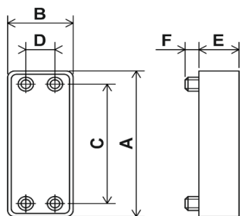
Rozmerová schéma
