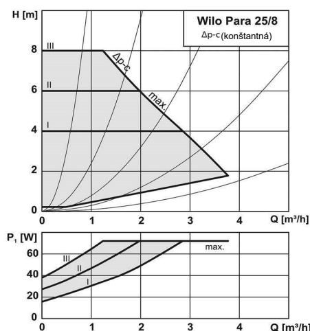
Charakteristiky Δp-c (konštantná)
