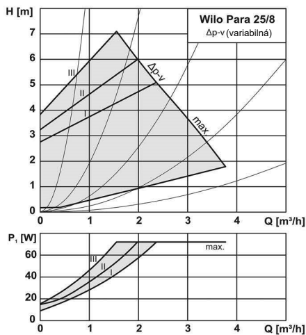
Charakteristiky Δp-v (variabilná)
