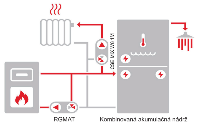
Príklad zapojenia II
