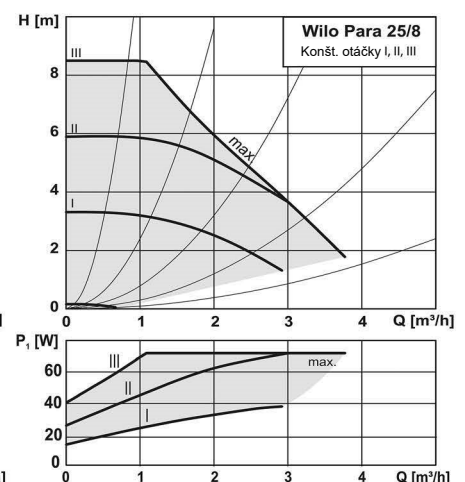
Charakteristiky n=konšt.
