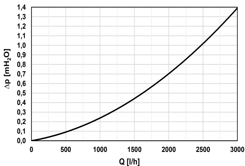
Graf tlakových ztrát
