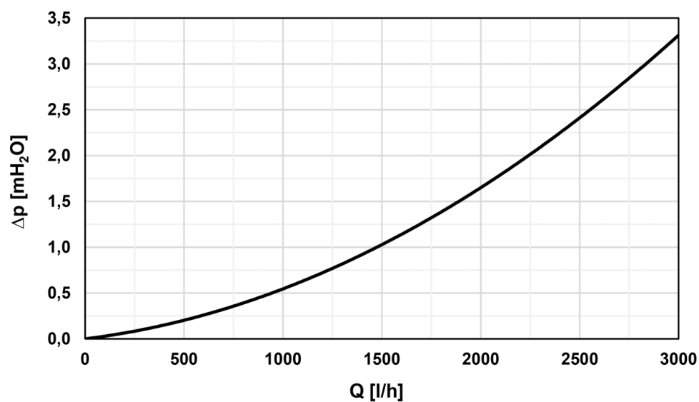
Graf tlakových ztrát
