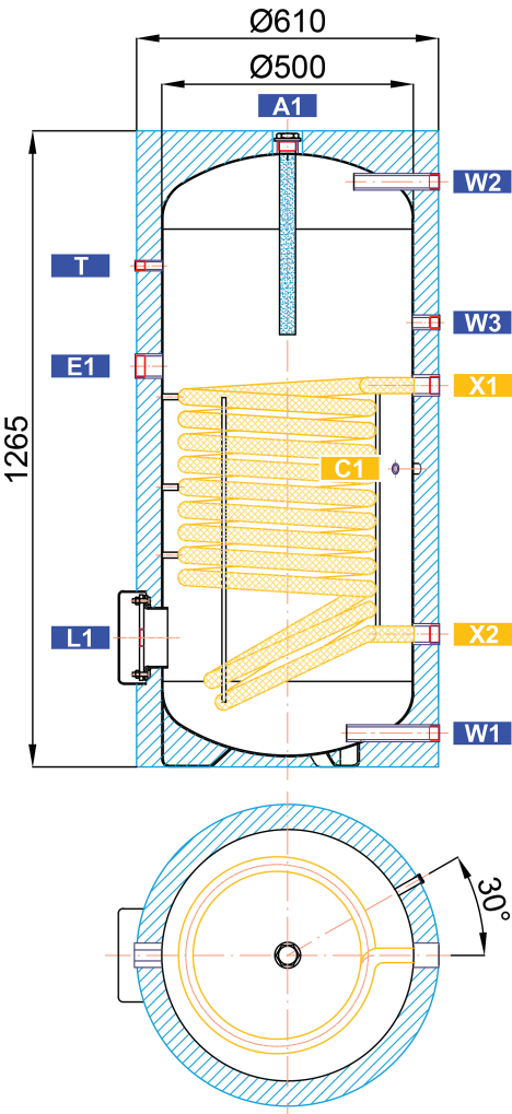
Rozměrové schéma
