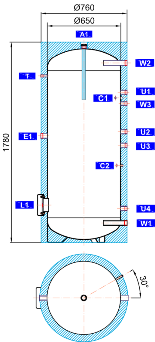
Rozměrové schéma
