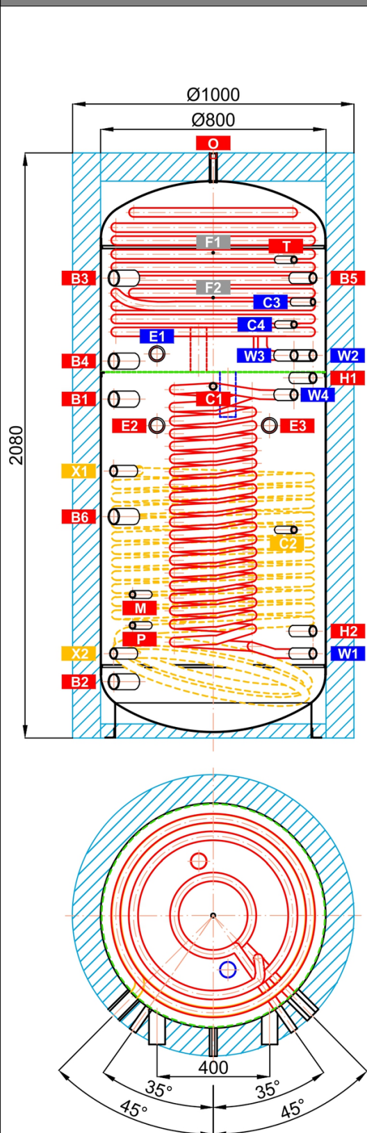
Rozměrové schéma
