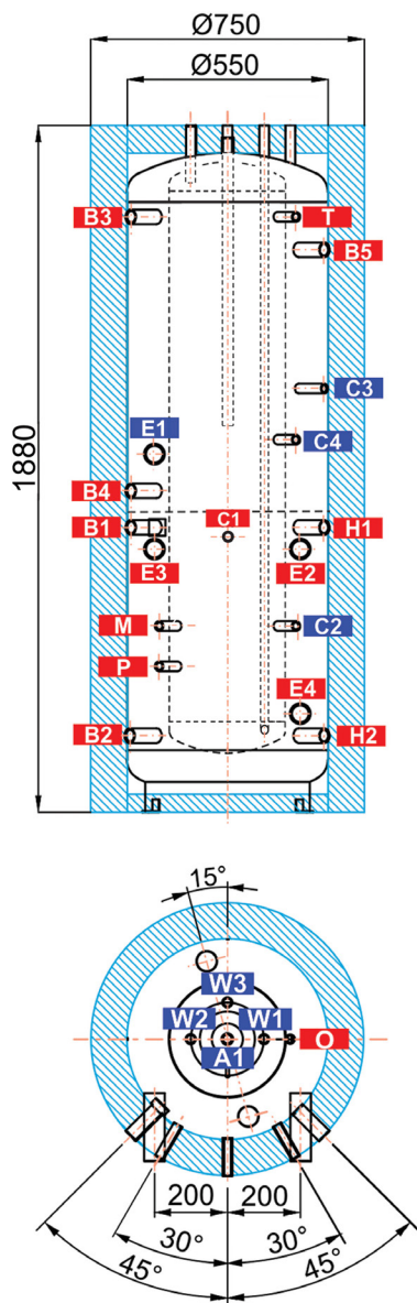
Rozměrové schéma
