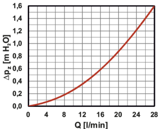
Průtokoměr 8-28 l/min
