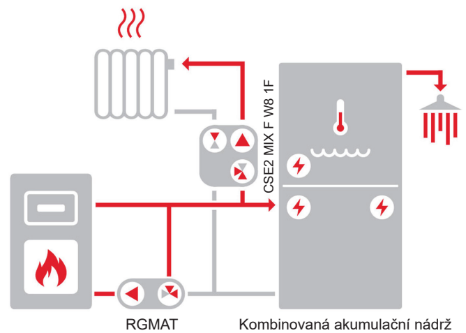
Příklad zapojení
