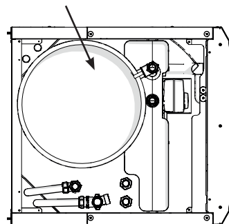
Horní připojení expanzní nádoby
