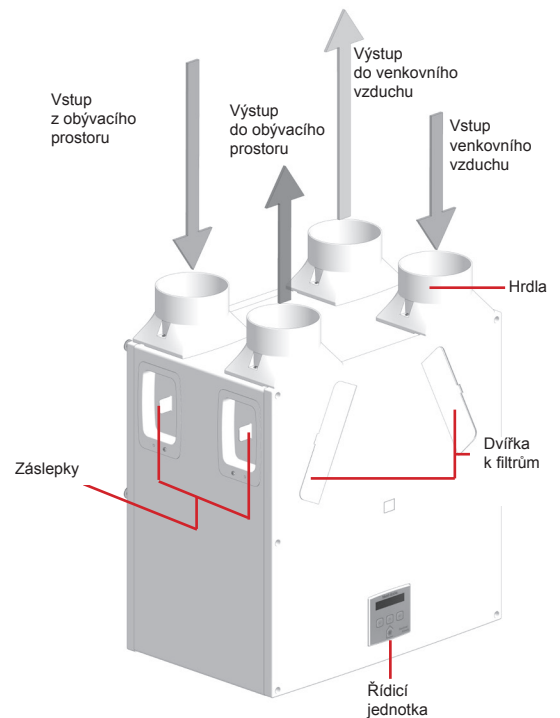
Obr. 1b: Sentinel Kinetic Plus - pohled na jednotku
