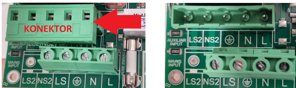
Obr. 22: Zapojení Ovládací fáze LS2
