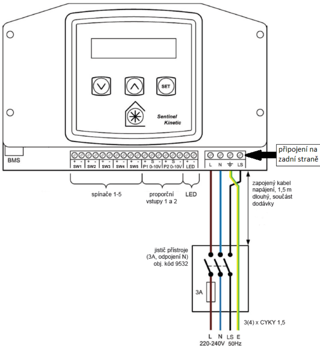
Obr. 21: Zapojení svorek
