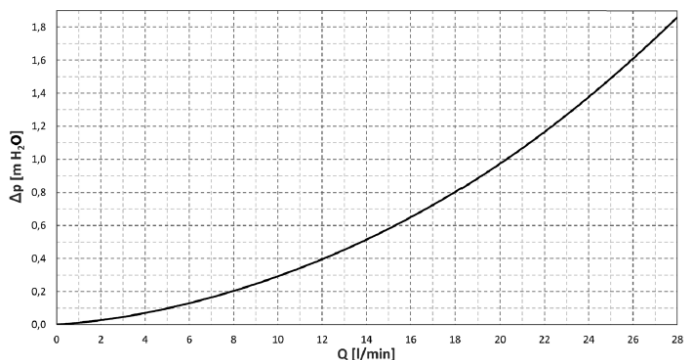
Připojení G 1" M – obj. kód 20577
